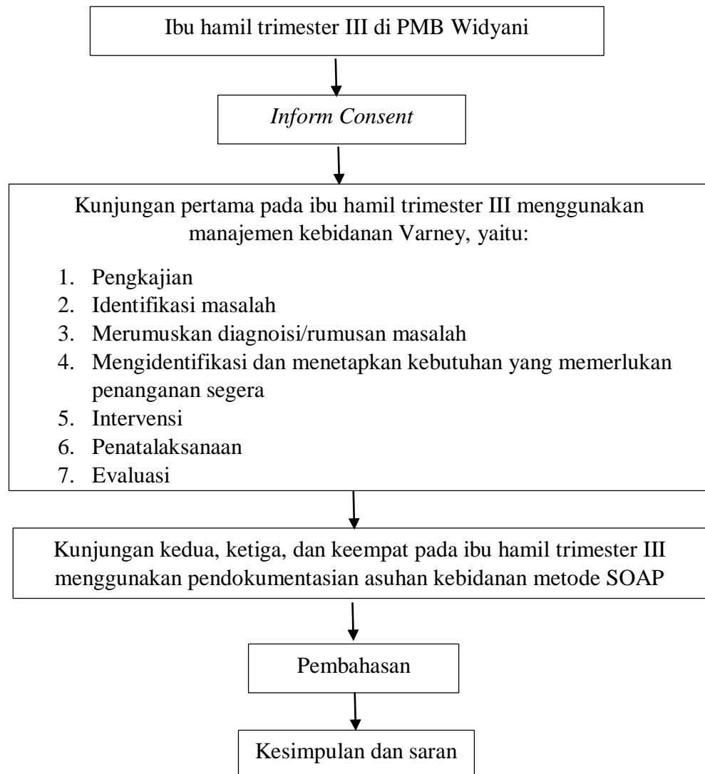
Gambar 3.1 kerangka kerja
